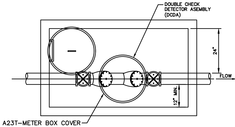
PLAN N.T.S.
